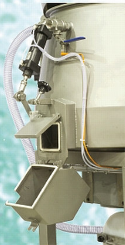
Geöffneter Auslass
