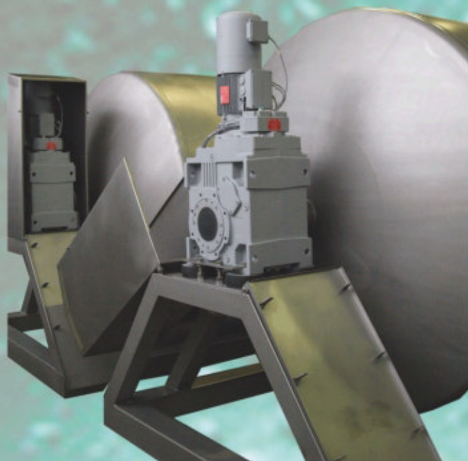
robustes Ölbadgeschmiertes Getriebe mit Verdeck
